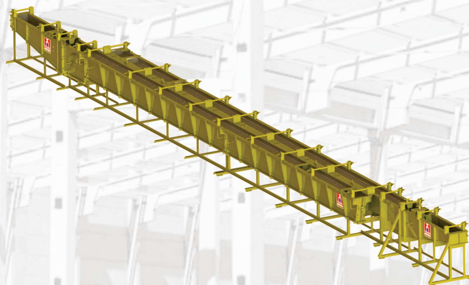
MOLDE VIGA T
