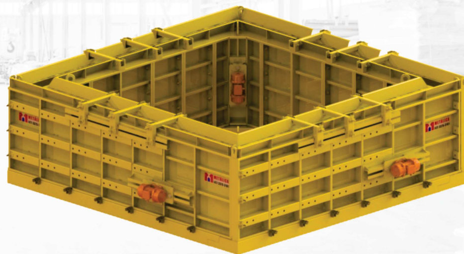
MOLDE GALERIA REGULÁVEL
