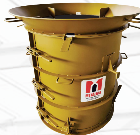
CONJUNTO VIBRATÓRIO
